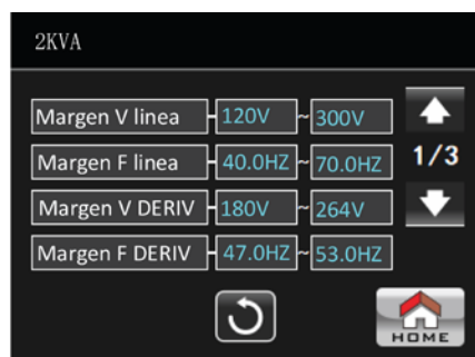
Información relativa a los parámetros - página 1
