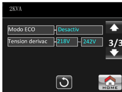
Configuración parámetros eléctricos - Página 3
