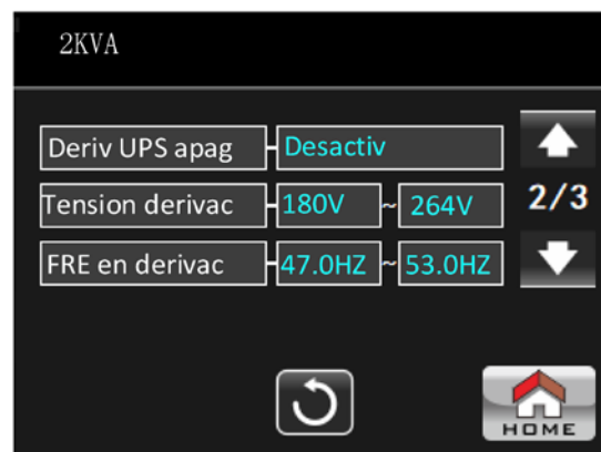
Configuración parámetros eléctricos - Página 2
