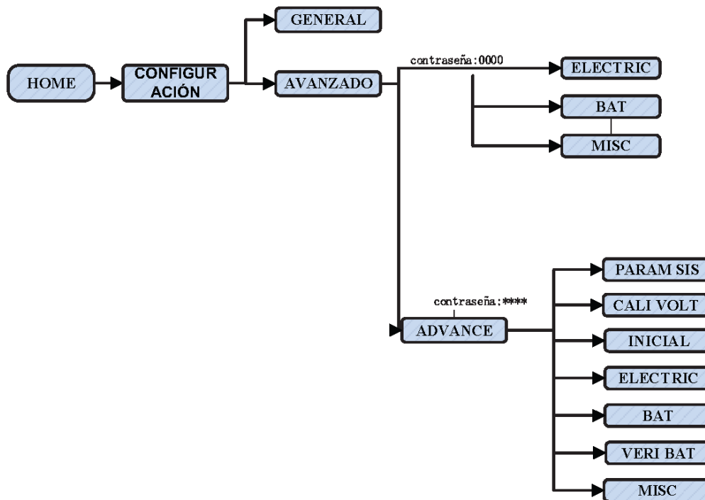
Jerarquía del menú
